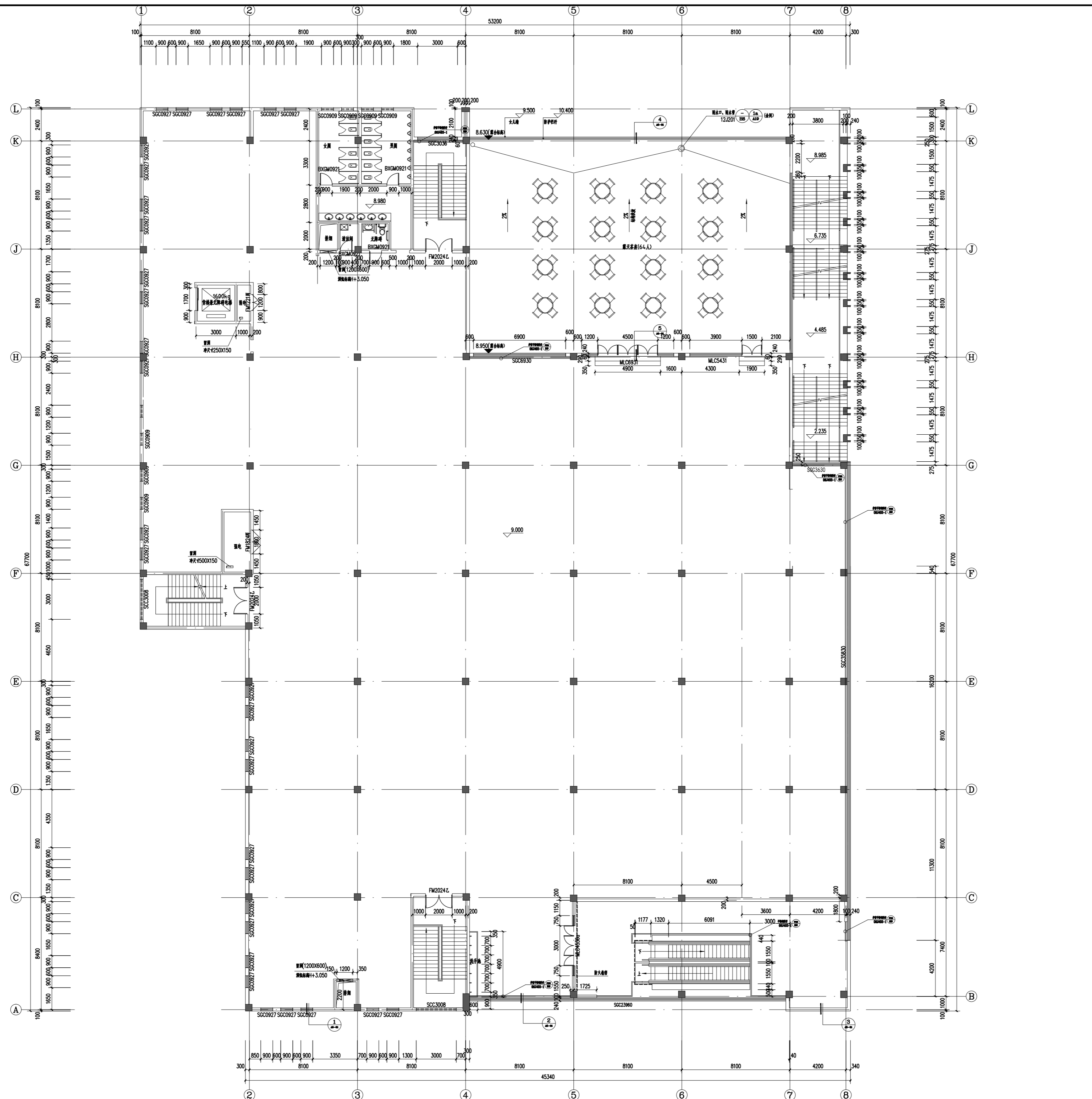
三层平面图 1:100 本层建筑面积2828.24㎡
